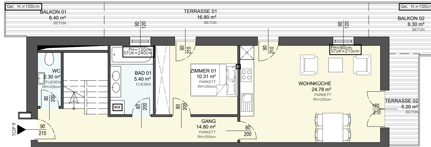
1. DACHGESCHOSS
