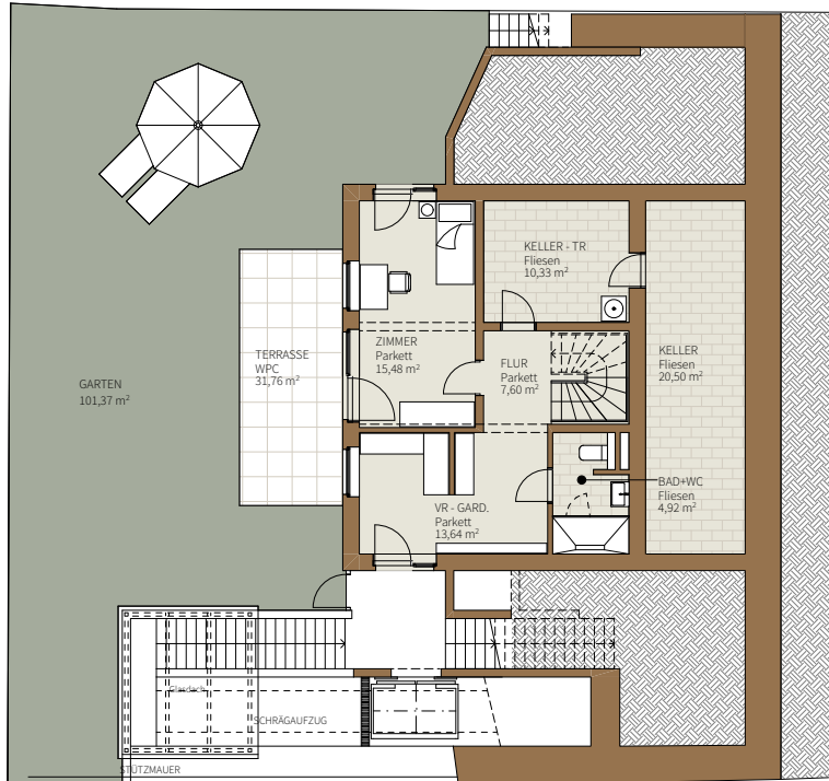
Ebene 1 HAUS 1 EG
