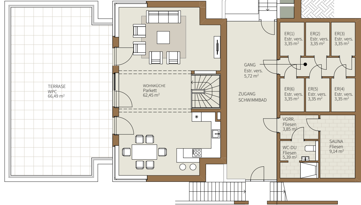
Ebene 6 HAUS 4 OG 2
