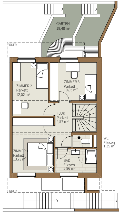
Ebene 5 HAUS 4 OG 1
