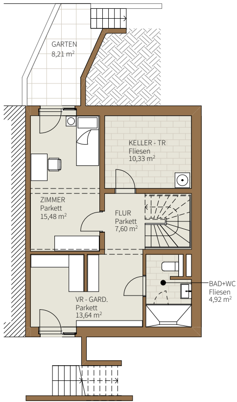
Ebene 4 HAUS 4 EG
